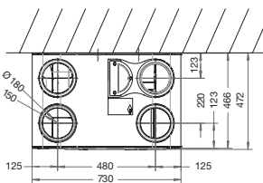
pohled shora – připojovací hrdla
