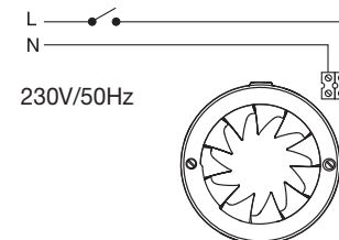
připojení ventilátoru k síti
