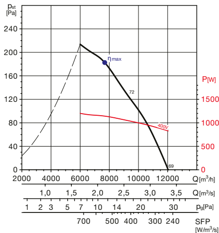
HXTR-TXTR/4-560
