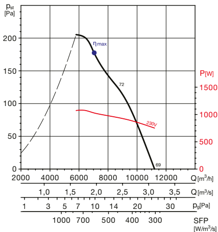
HXBR-TXBR/4-560
