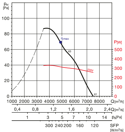
HXBR-TXBR/6-560
