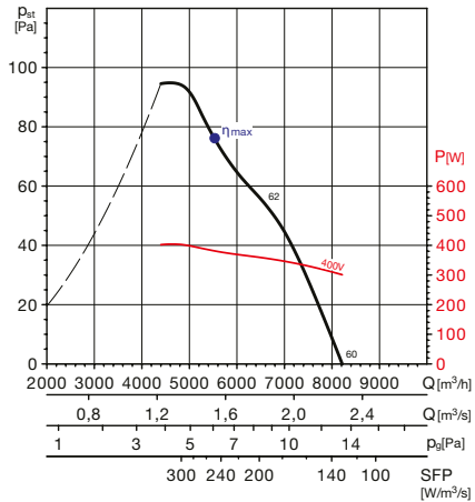
HXTR-TXTR/6-560
