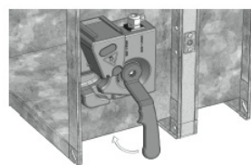
otevírací mechanismus
