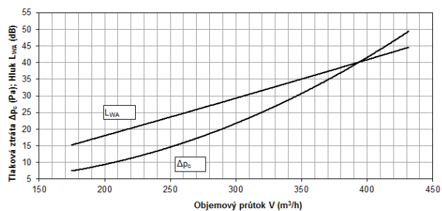
hluk, tlaková ztráta, průtok - VA C 500/24
