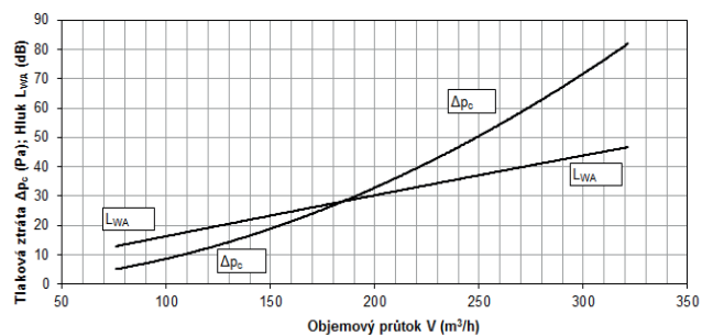
hluk, tlaková ztráta, průtok - VA C 400/16
