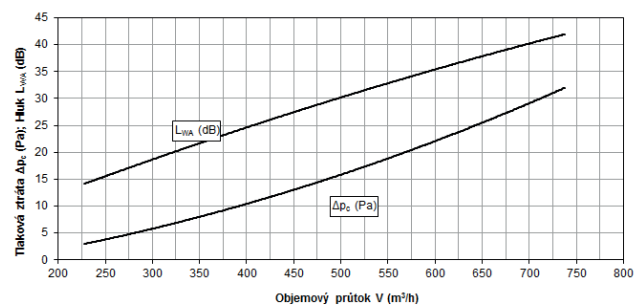
hluk, tlaková ztráta, průtok - VA C 600/48
