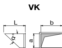
VK výfukový kus a \times b - \alpha^\circ - L
