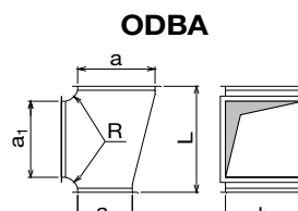
ODBA rozbočka šikmá a \times b - a_1 - a_2 - L - R
