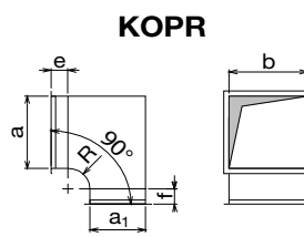
KOPR koleno přechodové a \times b - a_1 - R
