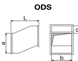
ODS odskok a \times b - o - L
