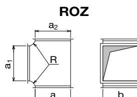
ROZ rozbočka a \times b - a_1 - a_2 - R
