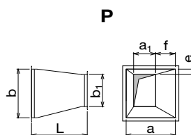
P přechod a \times b - a_1 \times b_1 - L
