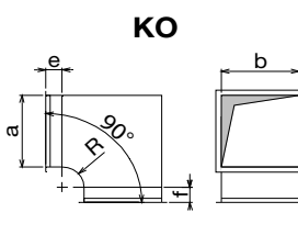
KO koleno a \times b - R
