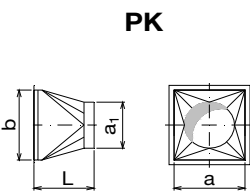
PK přechod na kruh a \times b - a_1 - L
