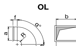
OL oblouk a \times b - \alpha^\circ - R
