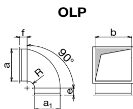
OLP oblouk přechodový a \times b - a_1 - R
